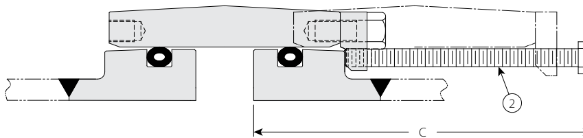
膨胀节接头现场拆卸空间要求
