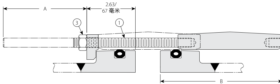
膨胀节接头现场装配空间要求
