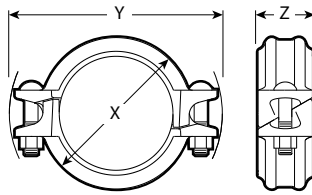
Dimensions 1 ½ – 4\"/>
