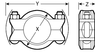
5 – Dimensions 12\"/>
