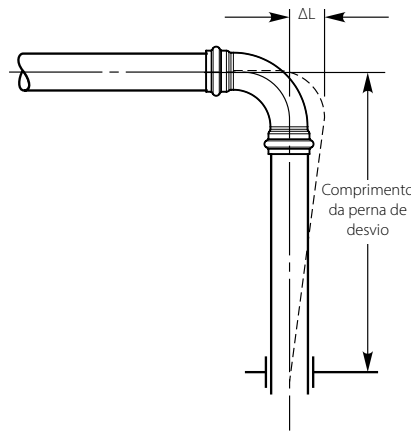
Compensador de expansão “Curva em L” Figura 1
