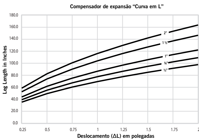
Compensador de expansão “Curva em L” Figura 1
