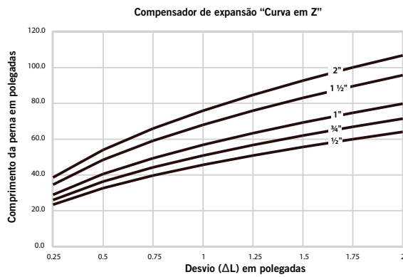
Compensador de expansão "Curva em Z"
