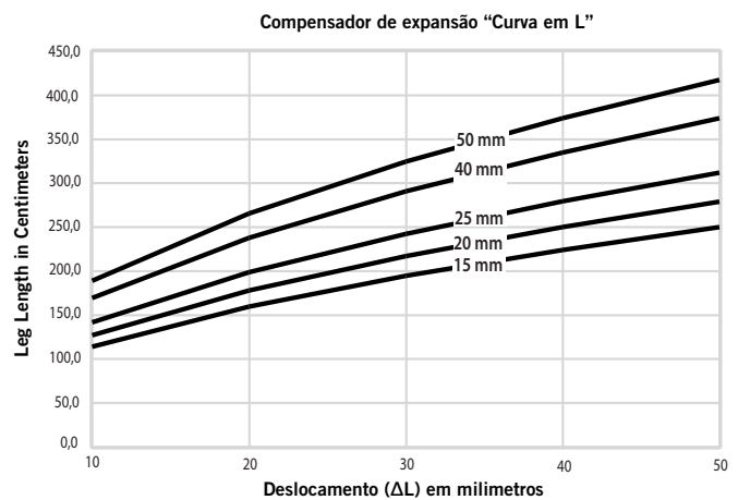
Compensador de expansão “Curva em L” Figura 1
