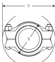
Połączenie zmontowane typu 905
