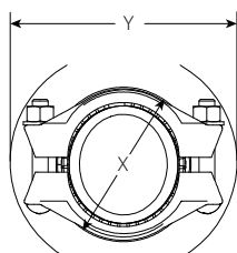
Wstępnie zmontowany typu 905 (gotowy do montażu)
