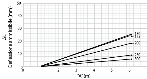
Movimento StrenghThin™ 100 - "spesso" 6 - 12"/DN150 - DN300: Spessore della parete > 3,1 mm
