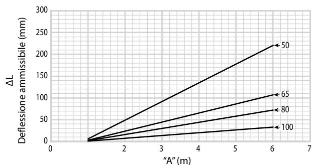
Movimento StrenghThin™ 100 - "spesso" 2 - 4"/DN50 - DN100: Spessore della parete > 2,3 mm
