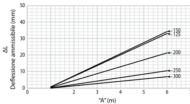
Movimento di StrenghThin™ 100 - "sottile" 6 - 12"/DN150 - DN300: Spessore della parete ≤ 3,1 mm
