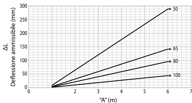
Movimento di StrenghThin™ 100 - "sottile" 2 - 4"/DN50 - DN100: Spessore della parete ≤ 2,3 mm
