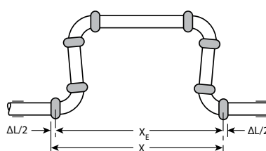
Figura 3 Dilatazione termica La tubazione cresce nell'anello - l'anello si contrae
