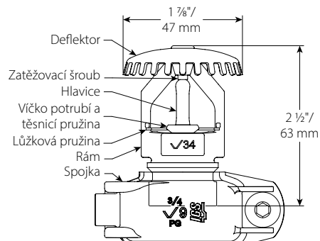
Drážka V3403
