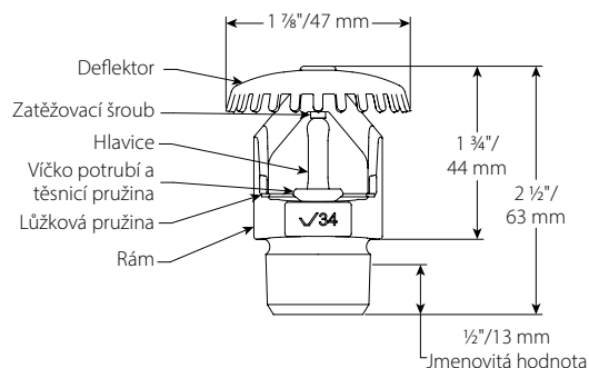
Závit V3403
