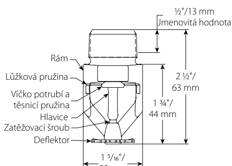
Závit V3407
