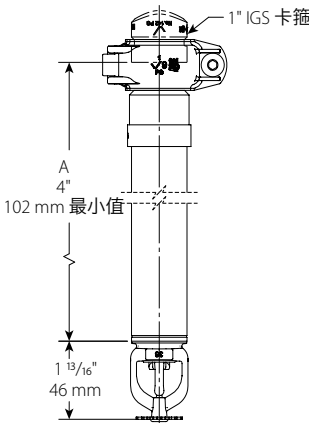
普通式带沟槽 V3613, V3615
