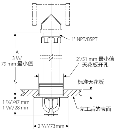
货架内置式带螺纹 V3613, V3615
