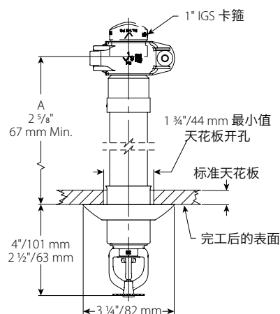
外伸裙座式带沟槽 V3613, V3615
