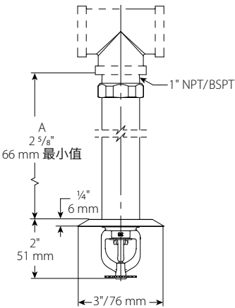
嵌入式带螺纹 V3613, V3615
