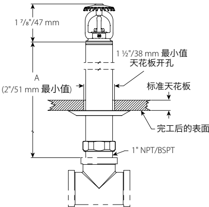
安装尺寸, 螺纹式 V3601, V3603
