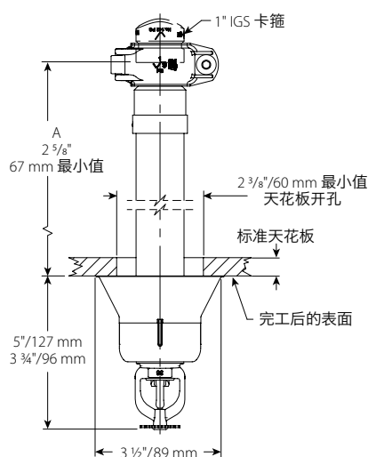
嵌入式带沟槽 V3613, V3615
