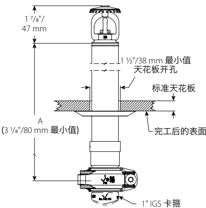
安装尺寸, 沟槽式 V3601, V3603
