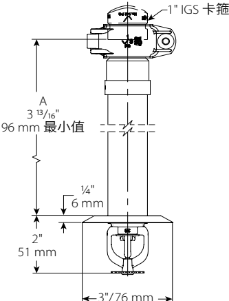
嵌入式带沟槽 V3613, V3615
