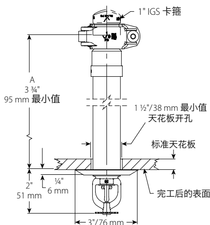
齐平式带沟槽 V3613, V3615
