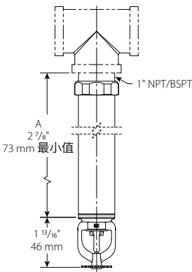
普通式带螺纹 V3613, V3615
