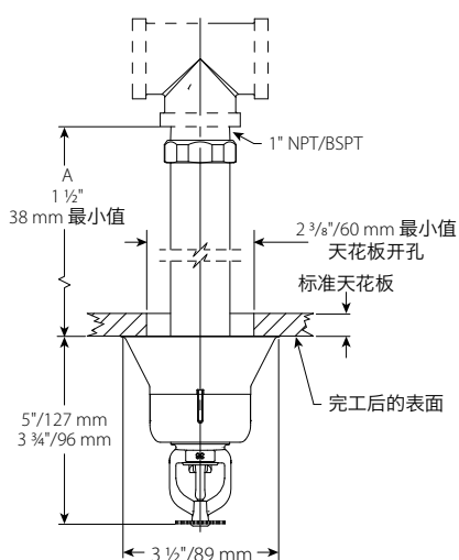
嵌入式带螺纹 V3613, V3615
