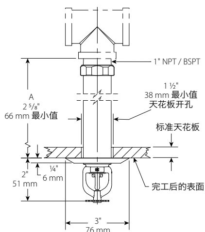
齐平式带螺纹 V3613, V3615
