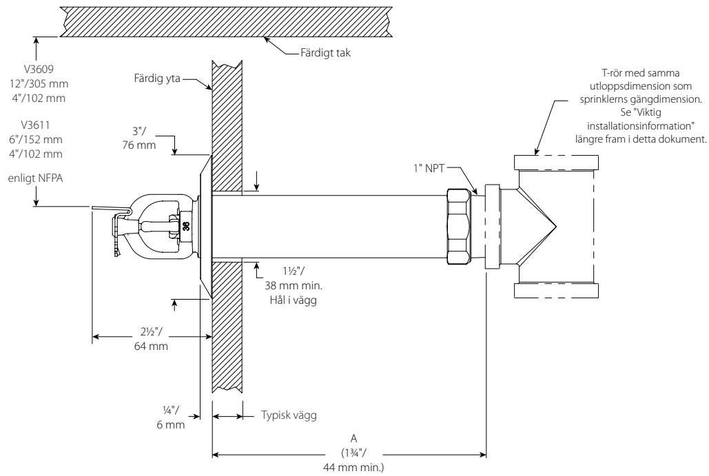
Försänkt, gängad V3609, V3611
