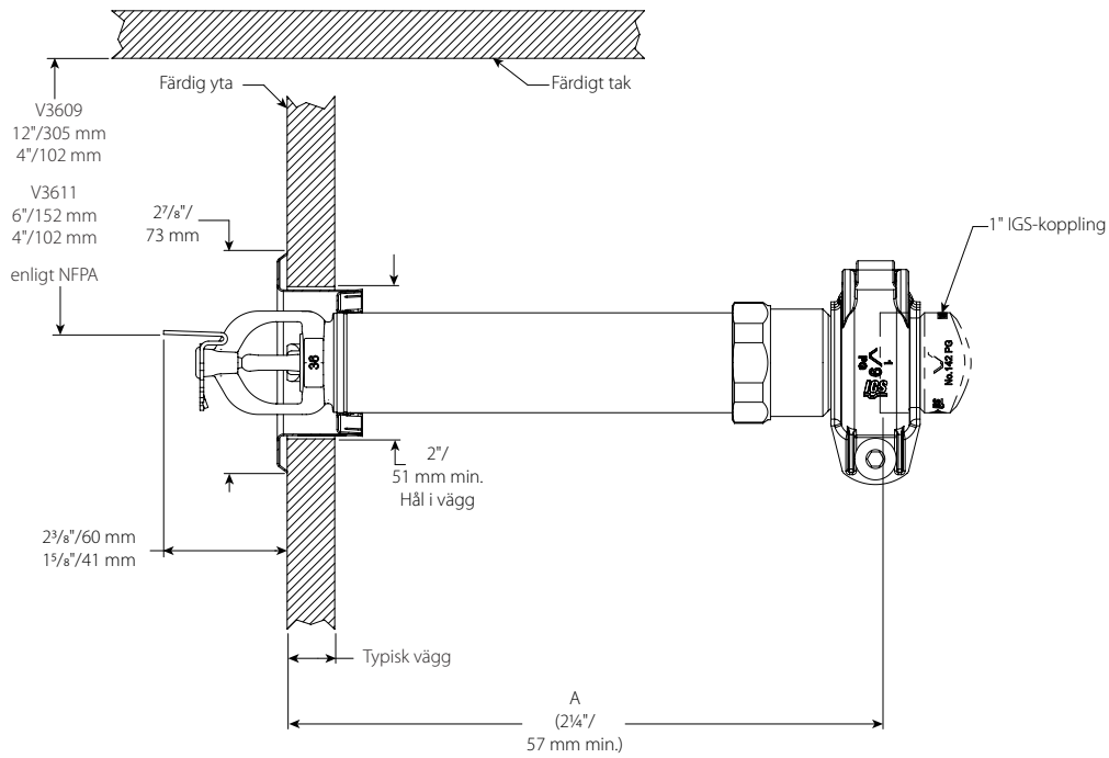
Infälld, rillad V3609, V3611
