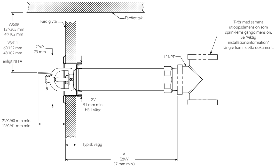
Infälld, gängad V3609, V3611
