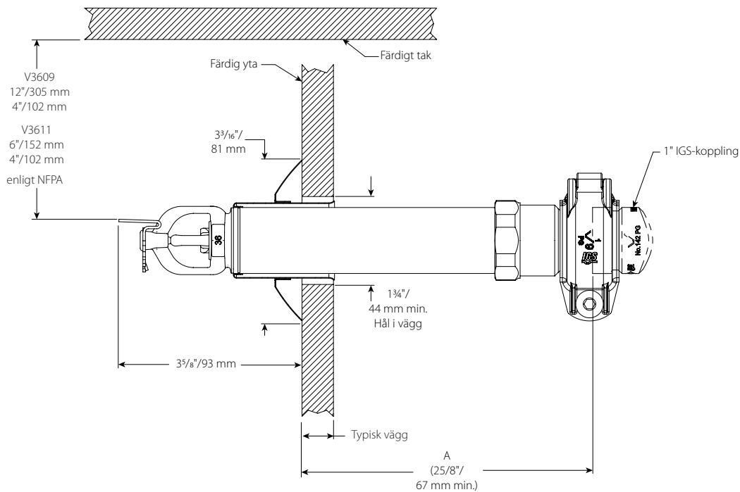
Hylsa och fläns, rillad V3609, V3611
