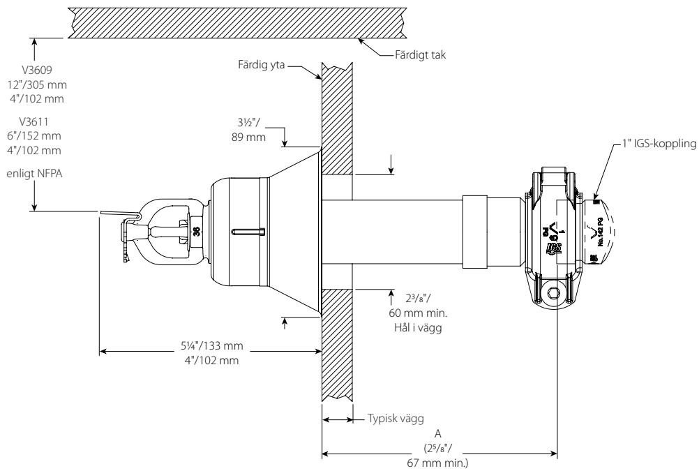
Förlängd, hylsa och fläns, rillad V3609, V3611
