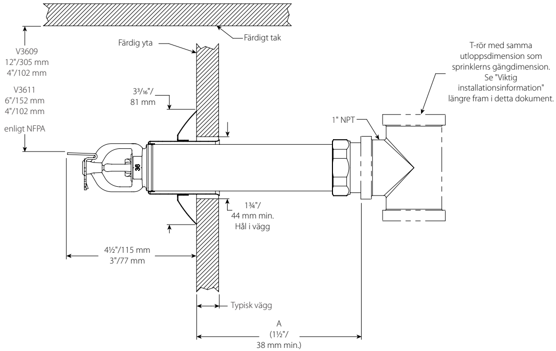
Hylsa och fläns, rillad V3609, V3611
