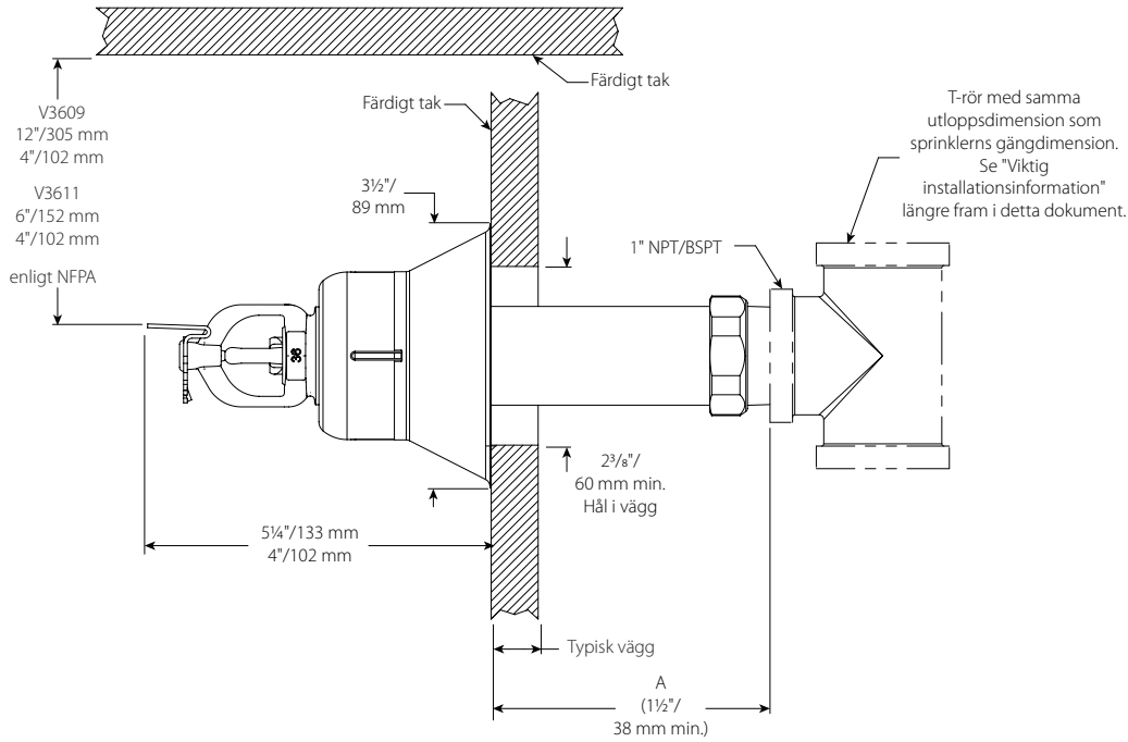
Förlängd, hylsa och fläns, gängad V3609, V3611
