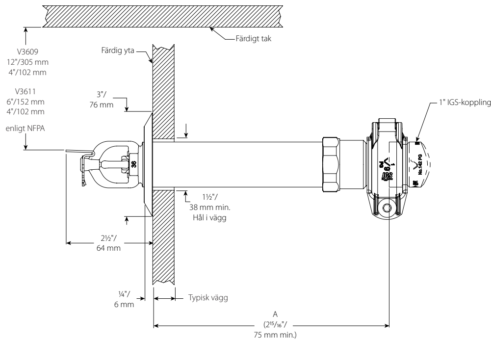
Försänkt, rillad V3609, V3611
