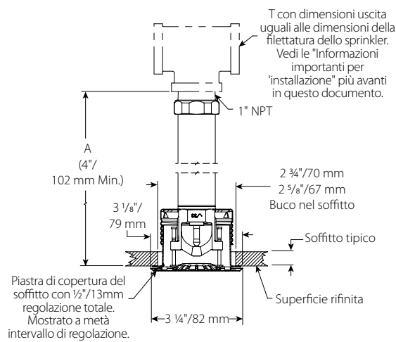
A sospensione nascosta, Filettata V3301, V3303
