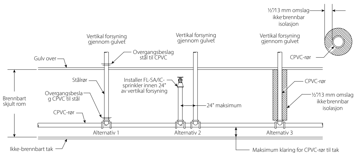
FIGUR 3 CPVC-RØR INSTALLERT SOM ET VERTIKALT STIGERØR (TVERRSNITTVISNING)
