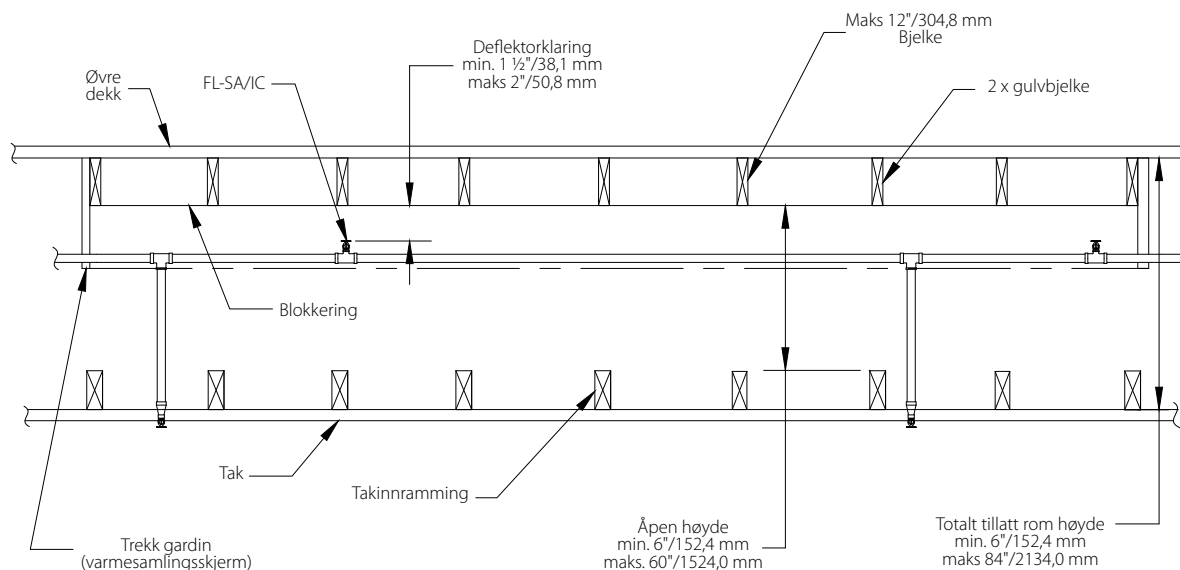
FIGUR 4 SOLID TREBJELKEKONSTRUKSJON MED INTEGRERT STÅLRØR (TVERRSNITTVISNING)
