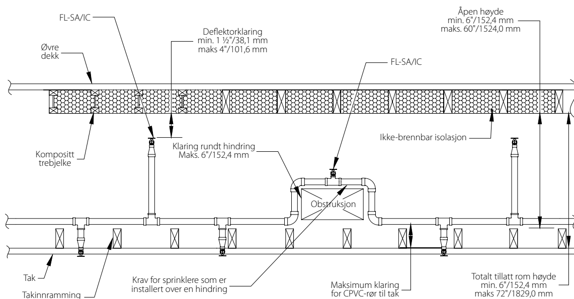
FIGUR 2 SOLIDE ELLER KOMPOSITTE TREBJELKEKONSTRUKSJONER MED CPVC-RØR DER ØVRE DEKK ER FYLT MED IKKE-BRENNBAR ISOLASJON (TVERRSNITTVISNING)
