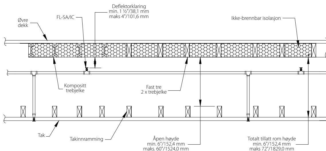
FIGUR 5 SOLIDE TREBJELKEKONSTRUKSJONER MED INTEGRERT STÅLRØR UTEN ISOASJON ELLER KOMPOSITTREBJELKEKONSTRUKSJONER MED INTEGRERT STÅLRØR DER ØVRE DEKK ER FYLT MED IKKE-BRENNBAR ISOLASJON (TVERRSNITTVISNING)
