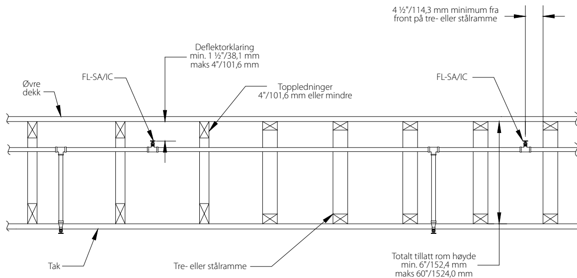
FIGUR 6 UHINDRET ÅPEN RAMMEKONSTRUKSJON I TRE OG STÅL MED INTEGRERT STÅLRØR (TVERRSNITTSVISNING)
