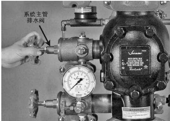
1. 开启系统主管排水阀。确认系统已排干积水。
