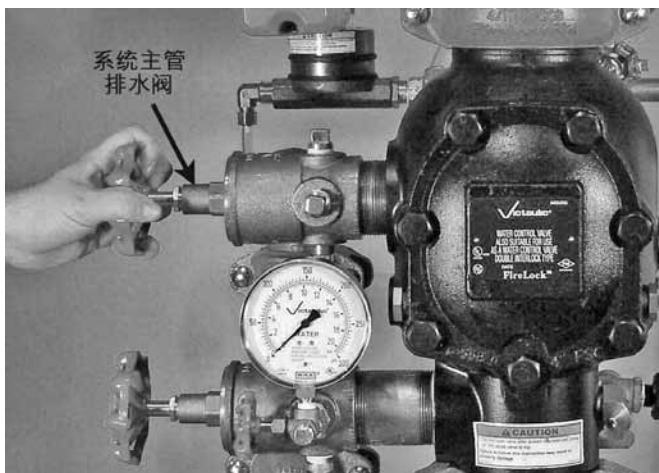
8. 打开系统主管排水阀，排出所有积水，并释放系统气压。
