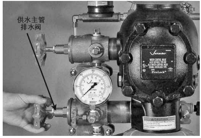
12. 打开供水主管排水阀。
