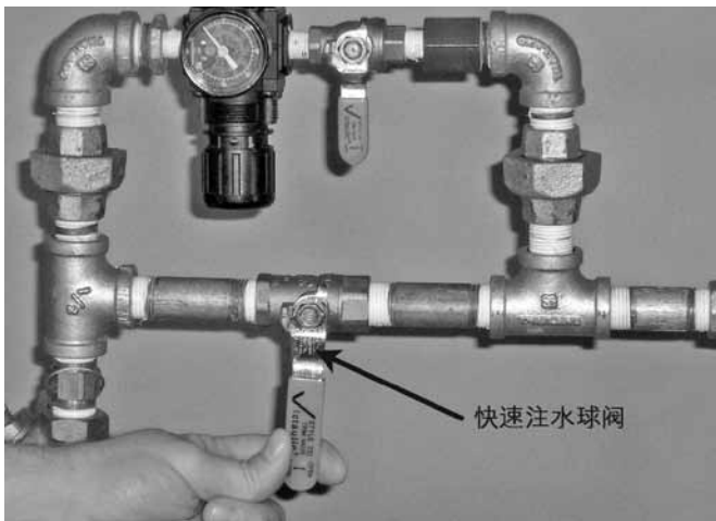
10. 对于气动(干式先导)释放系统: 达到系统正常气压后, 请关闭AMTA上的快充球阀。
