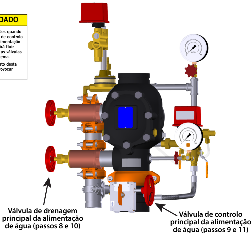
Trim de libertação pneumática (piloto seco) ilustrado (estação de acionamento manual não ilustrada para visibilidade dos componentes)
