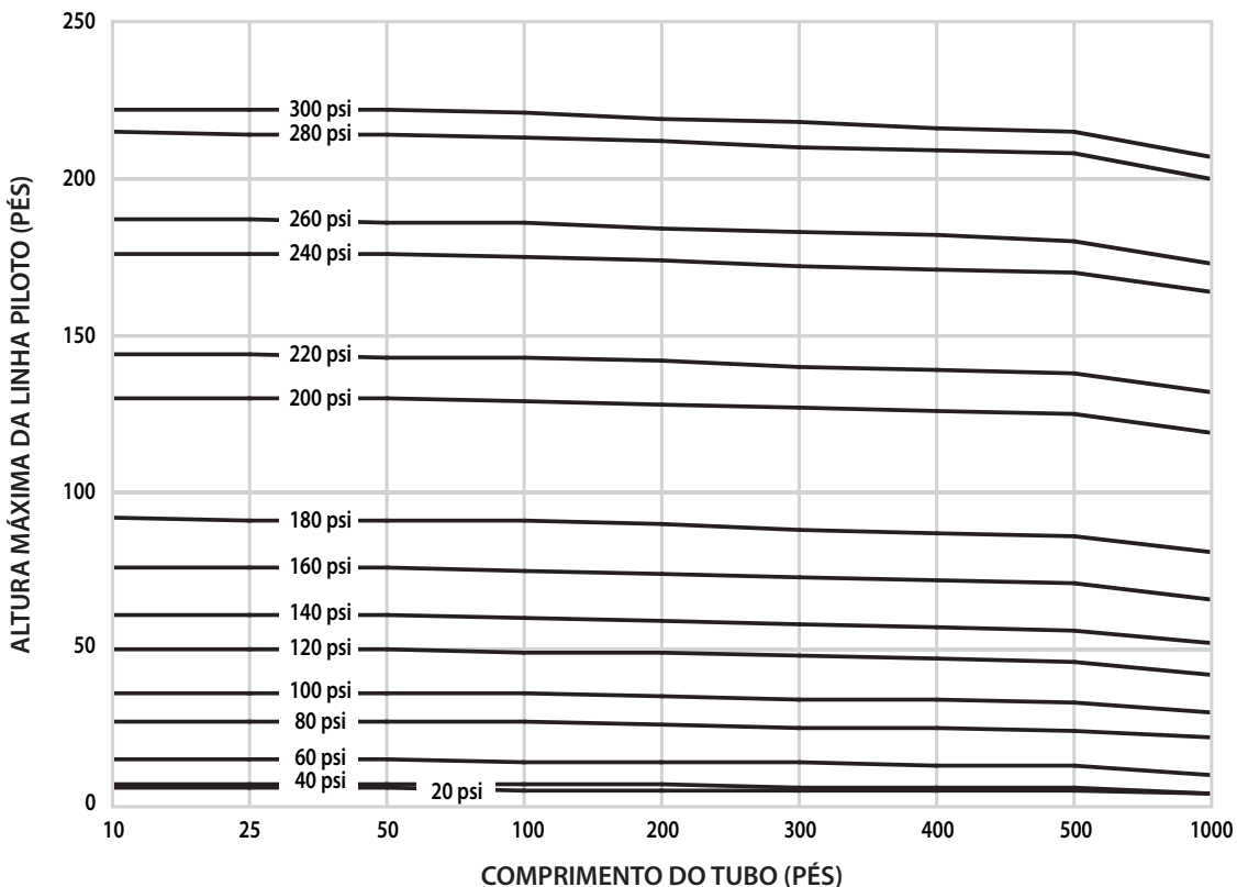
Válvula de tamanho de 6 pol./168,3 mm (inclui 165,1 mm)
