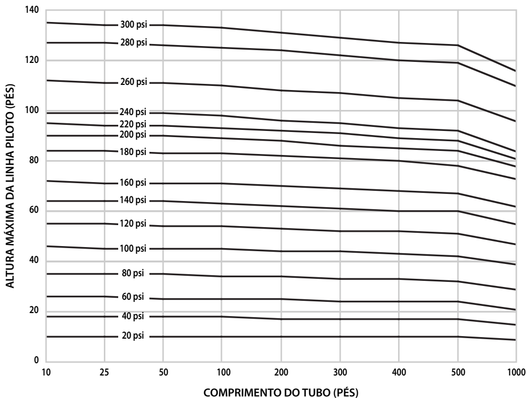
Válvula de tamanho de 4 pol./114,3 mm
