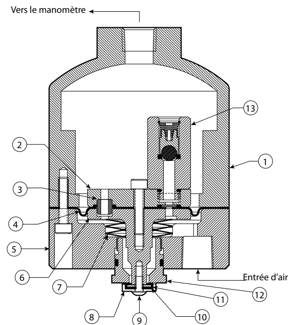
VUE EN COUPE AVEC CHAMBRE SUPÉRIEURE TOURNÉE DE 45° ET BOULON ENLEVÉ POUR PLUS DE CLARTÉ
