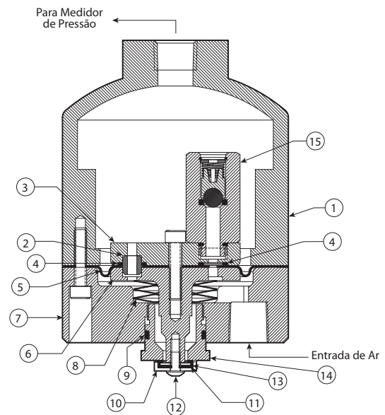
SEÇÃO TRANSVERSAL COM A CÂMARA SUPERIOR GIRADA EM 45° E O PARAFUSO REMOVIDO PARA MAIOR CLAREZA Exagerado para proporcionar clareza
