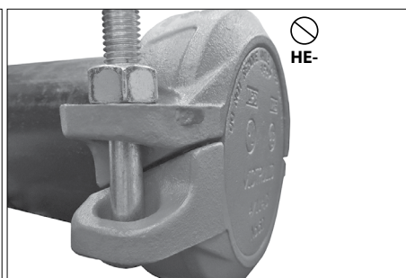
HELYTELEN ÖSSZESZERELÉS (A CSAVARTARTÓ VÁLLAK NINCSENEK FÉM-FÉM ÉRINTKEZÉSBE)
