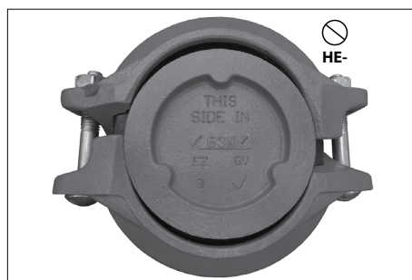
HELYTELEN ÖSSZESZERELÉS (A ZÁRÓSAPKA NEM MEGFELELŐ OLDALA VAN FELFELÉ - AZ ELEMET NEM LEHET MEGHÚZNI, HOGY A CSAVARTARTÓ VÁLLAK FÉM-FÉM ÉRINTKEZÉSBE KERÜLJENEK)
