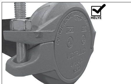
HELYES ÖSSZESZERELÉS (A ZÁRÓSAPKA A KUPLUNGBAN BELÜL VAN, A MEGFELELŐ OLDALLAL FELFELÉ ÉS A KUPLUNG CSAVARTARTÓ VÁLLAK FÉM-FÉM ÉRINTKEZÉSBE VANNAK)
