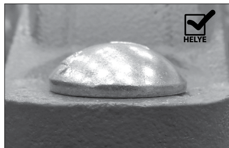
HELYES CSAVAR ILLESZKEDÉS (MINDEN EGYES CSAVAR OVÁLIS NYAKA MEGFELELŐEN ILLESZKEDIK A CSAVAR LYUKÁBA)
