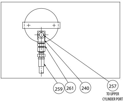
VIEW A-A
